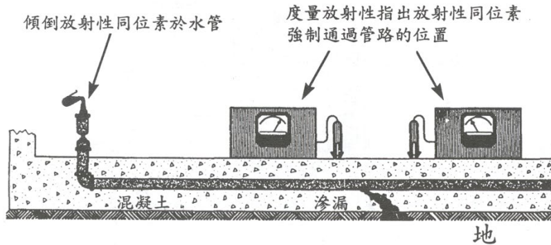
圖 4 測漏計
